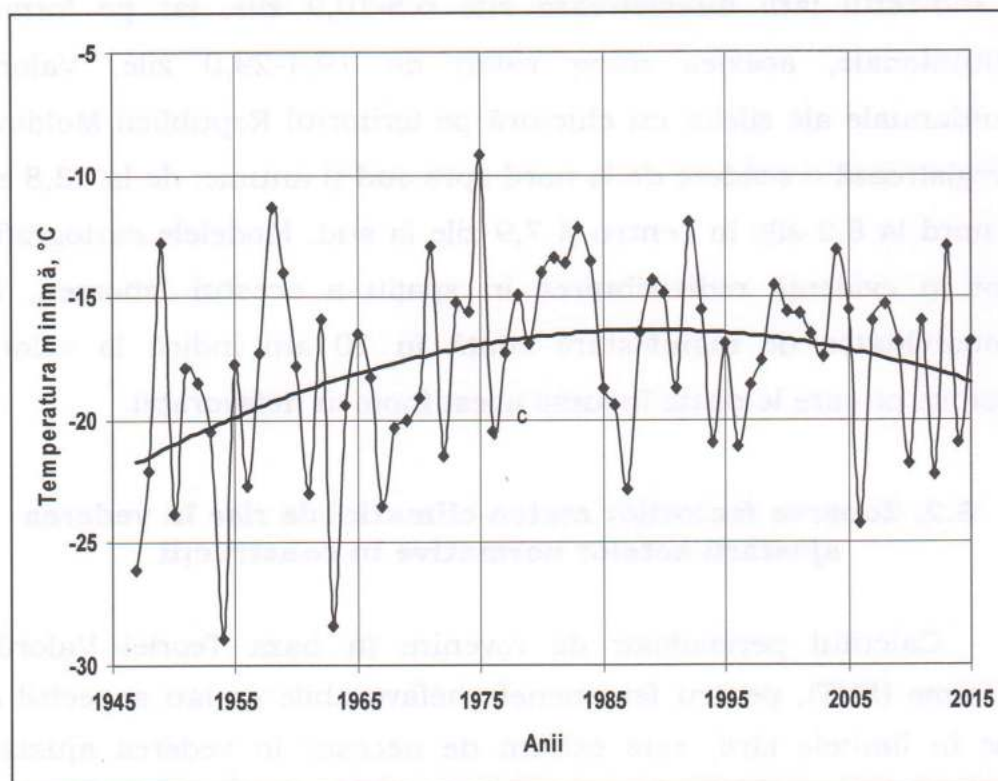
Fig.3.2.1. Temperaturile minime anuale (1946-2015), st.Chişinău
