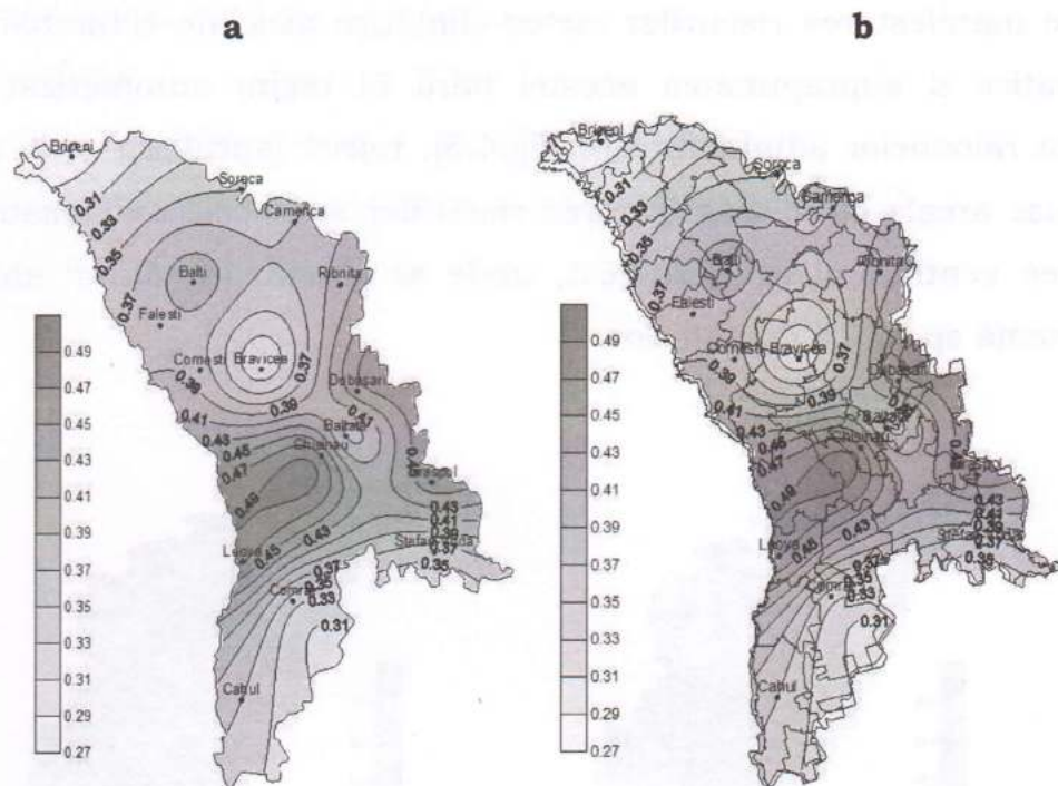
Fig.4.4. Deviața standard a cantității anuale a precipitațiilor atmosferice pe teritoriul Republicii Moldova (a- la nivel de țară; b- la nivel de raion administrativ)
