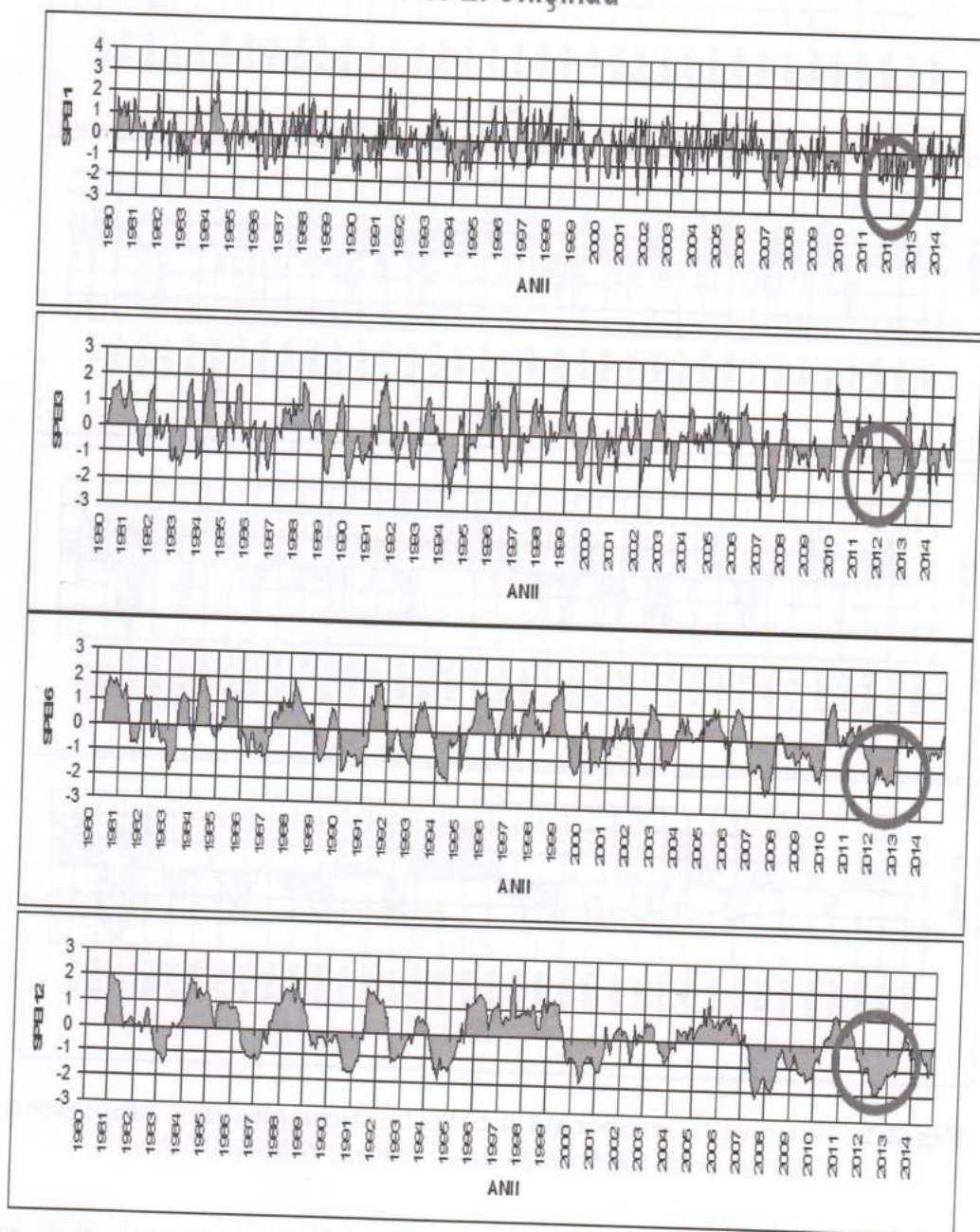
Fig.2.8. Estimarea temporală a SPEI în centrul țării (st. Chișinău) pentru diferite scări de timp (o lună; 3 luni; 6 luni; 12 luni)
