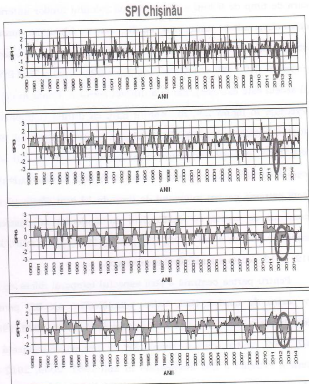
Fig.2.5. Estimarea temporală a SPI în centrul țării (st. Chișinău) pentru diferite scări de timp (o lună; 3 luni; 6 luni; 12 luni)
