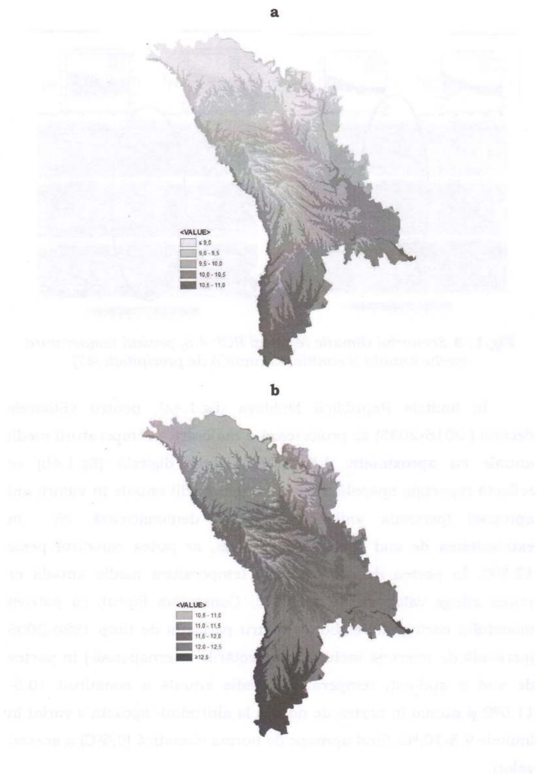
Fig.1.4. Modelarea cartografică a temperaturii medii anuale (a- 1986-2005; b- prognozată 2016-2035 cu RCP 4.5) pe teritoriul Republicii Moldova
