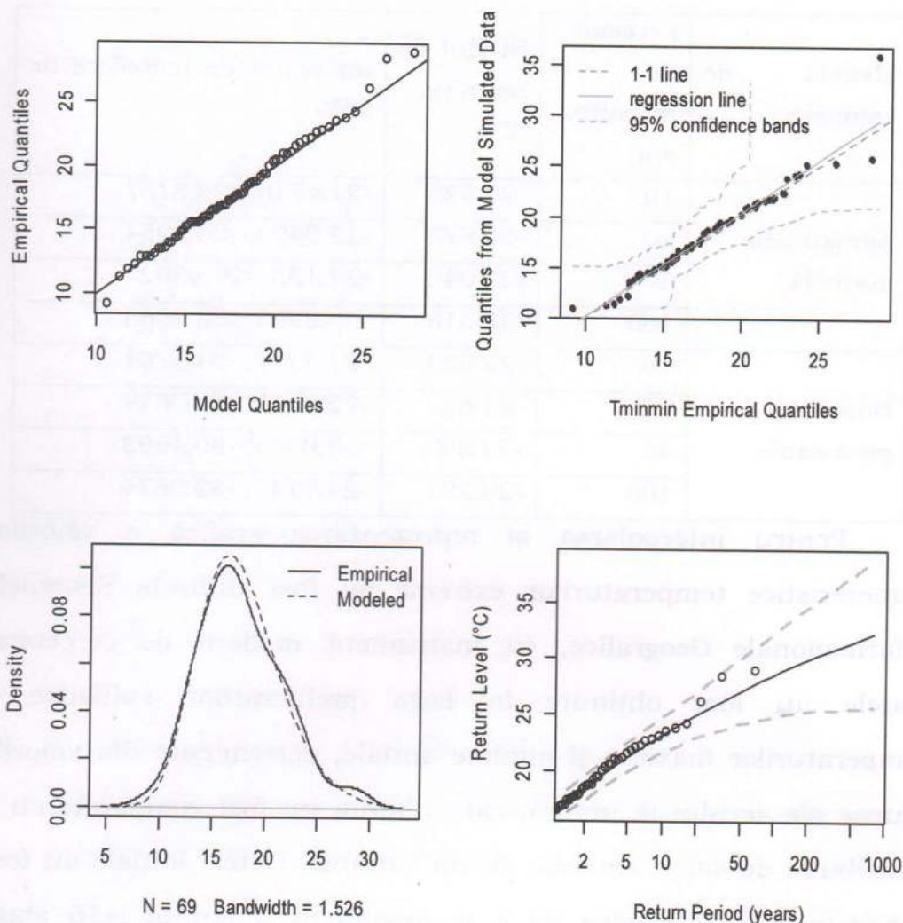
Fig.3.2.2. Perioada de revenire a temperaturilor minime (1946-2015), st.Chîșinău
