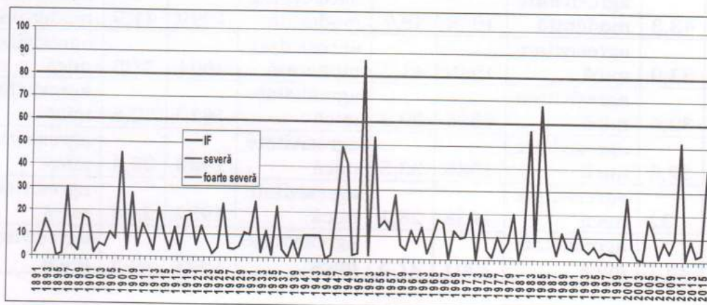
Fig.2.2.3. Dinamica Indicelui Fournier și agresivitatea pluvială (st. Chișinău, 1891-2016)
