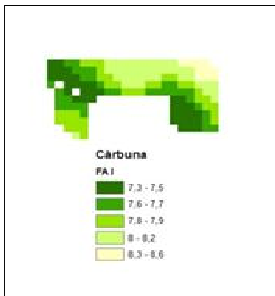
Figura 28. Distribuția spațială a valorilor Indicelui de Ariditate Forestier -FAI, calculat pentru Rezervația Peisajeră „Cărbuna”.
